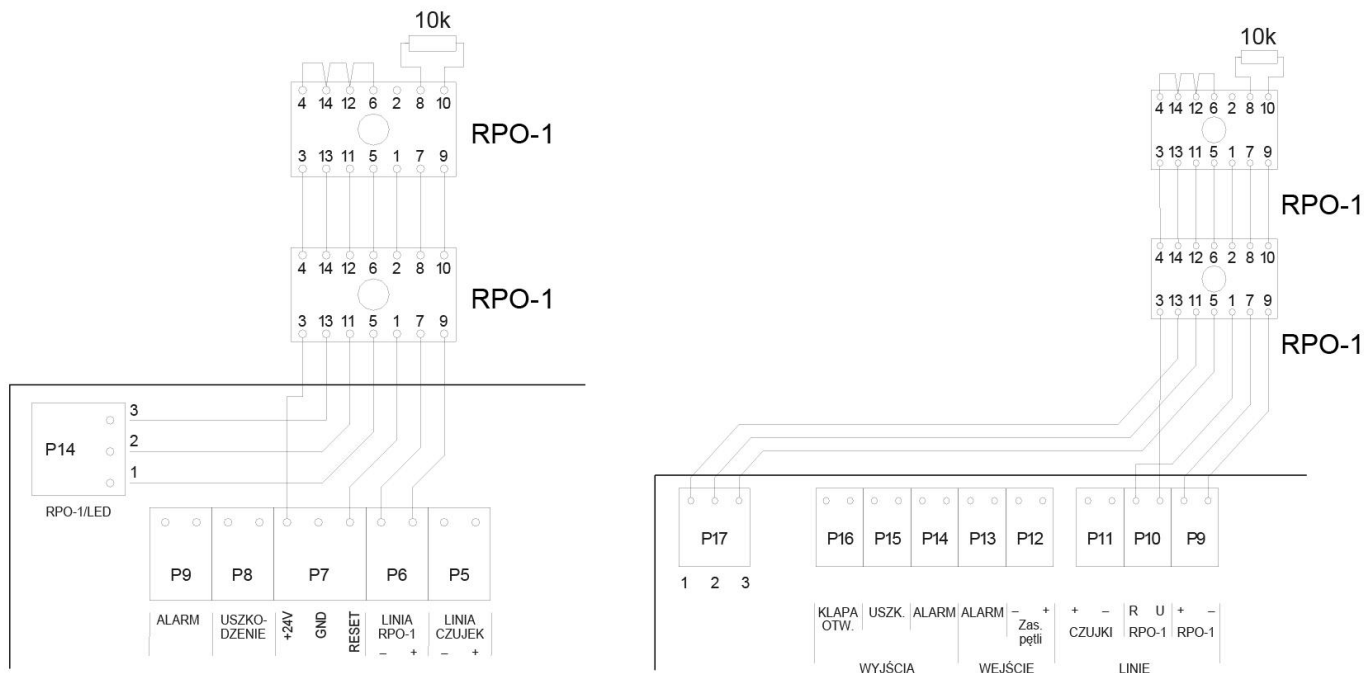
Rys.3. Schemat połączeń przycisku mcr RPO-1 z centralą mcr 0204 (po lewej) i mcr 9705 (po prawej).
